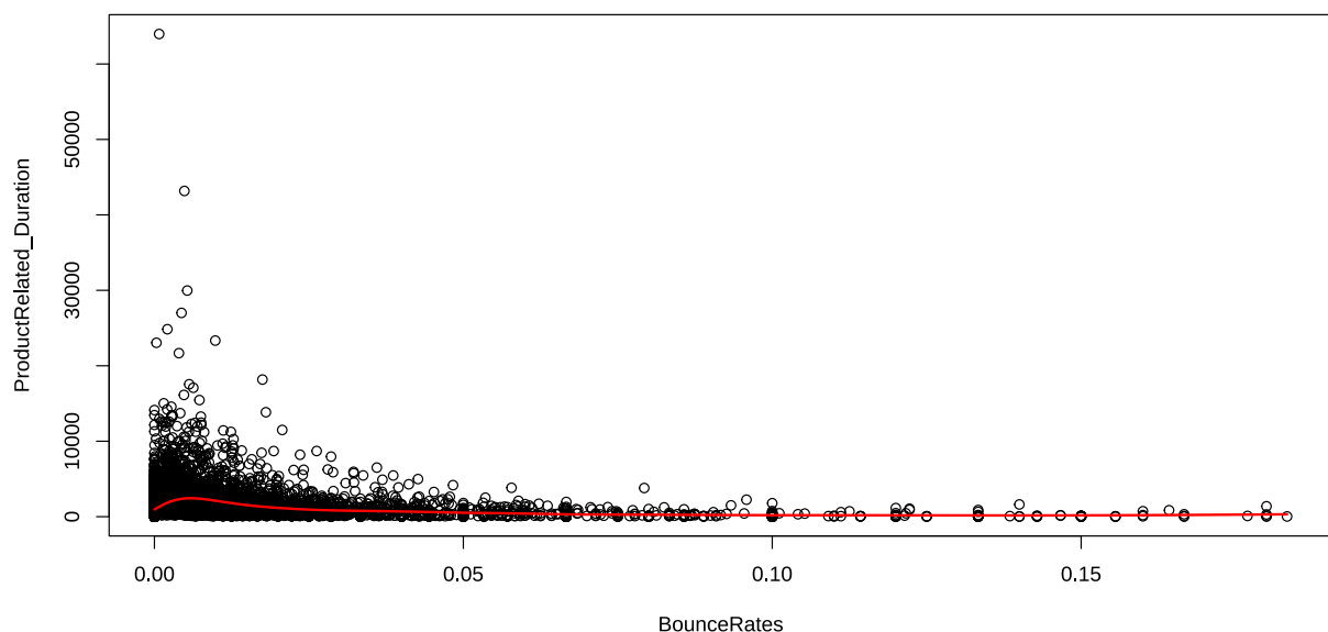
Glodaus spline modelio gerumo patikrinimas
