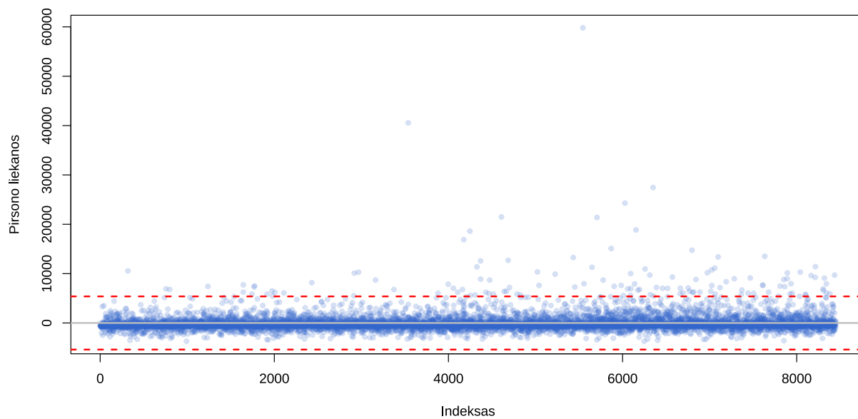
B-splainas: Pirsono liekanos
