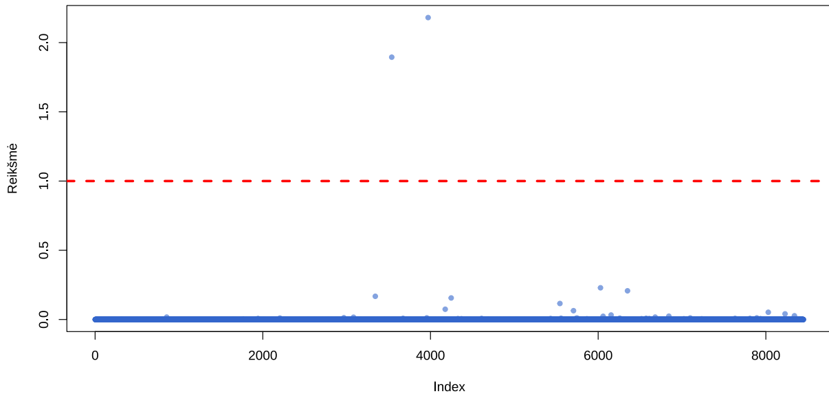
B-splainas: Kuko matas
