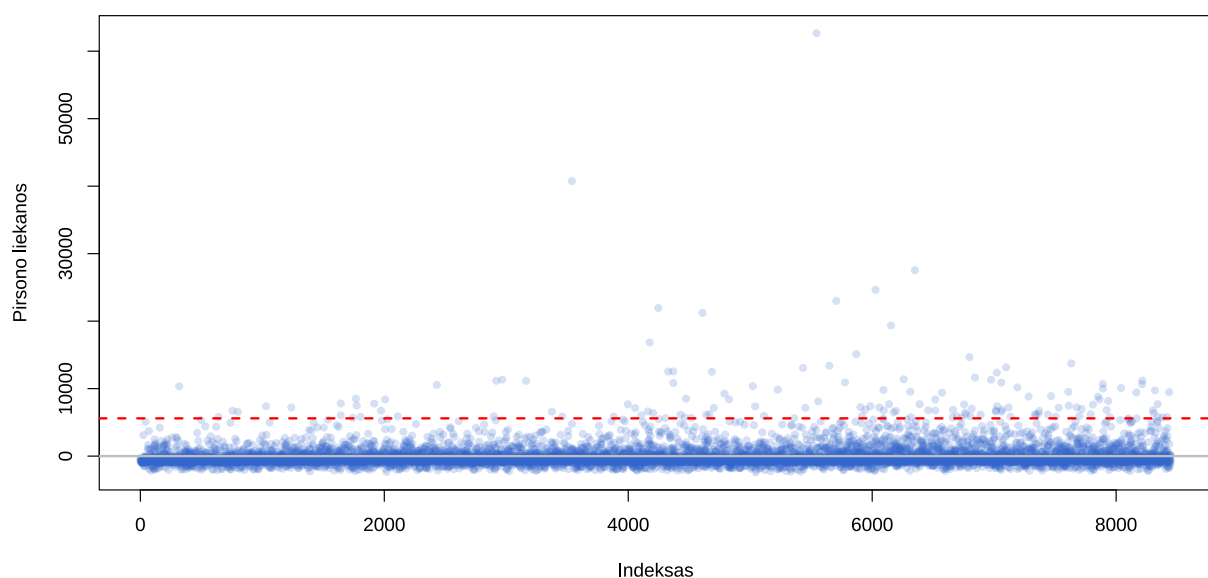
Glodusis splainas: Pirsono liekanos
